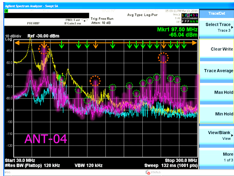
ANT-04の測定結果は電波暗室の結果に近い
